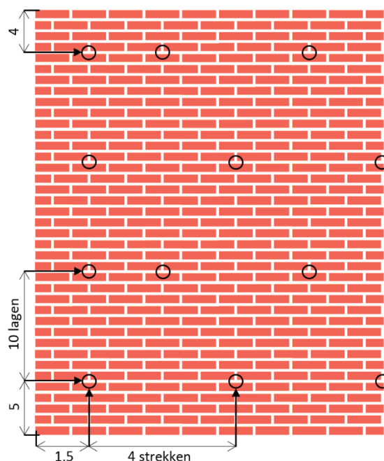
Figuur 5.2: Vulopeningen (waalformaat baksteen)
