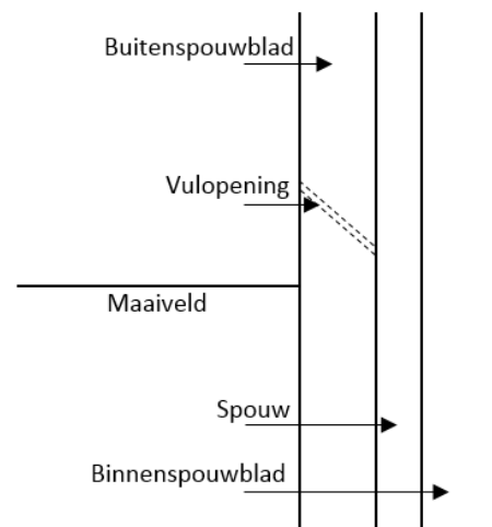
Figuur 5.4: Schuin boren
