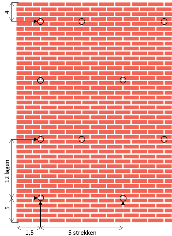
Figuur 5.2: Vulopeningen (waalformaat baksteen)
