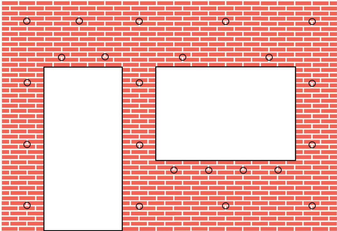
Figuur 5.3: Aangepast vulpatroon rond gevelopeningen
